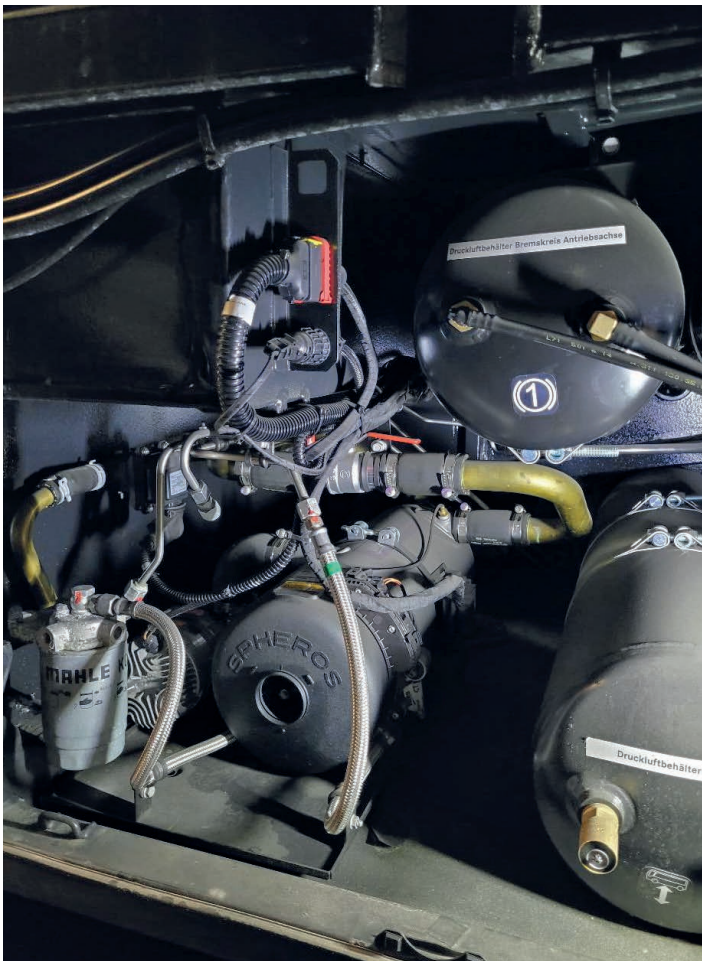
Einbausituation Thermo plus 300 CAN im Citaro LE B2E Bj. 2024.
