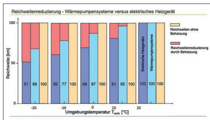
Vergleich: Reichweitenreduzierung beim Heizen mit elektrischem Heizgerät versus dem Heizen mit Wärmepumpe.
