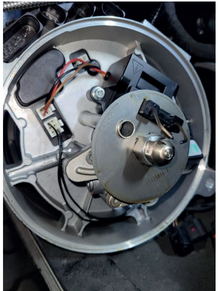
Geöffneter Brennerkopf einer Thermo plus 300 CAN nach einer Betriebszeit von 9 Monaten mit HVO 100 - frei von Ablagerungen.
